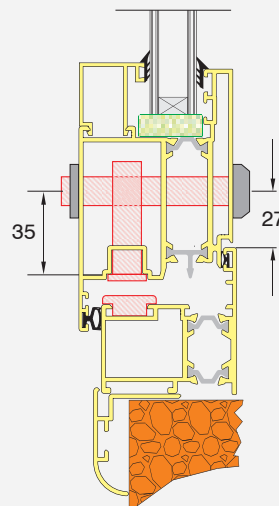
Opcional: Bisagras reforzadas
