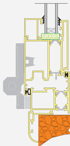
Opcional: Bisagras reforzadas
