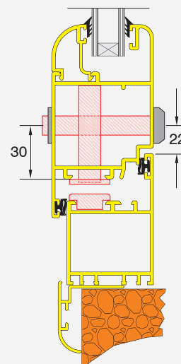
Opcional: Bisagras reforzadas
