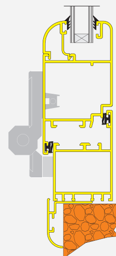
Opcional: Bisagras reforzadas
